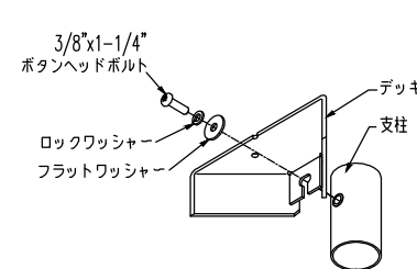
支柱とデッキ接続
