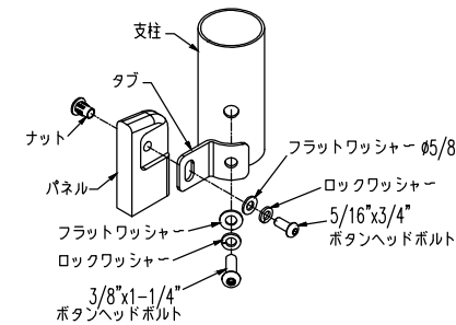
支柱と鋼管柵接続
