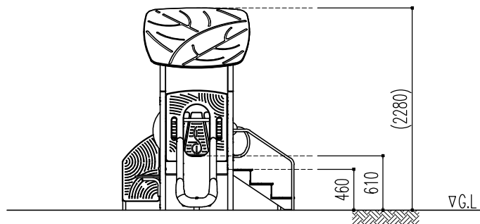
X立面図 S=1:60
