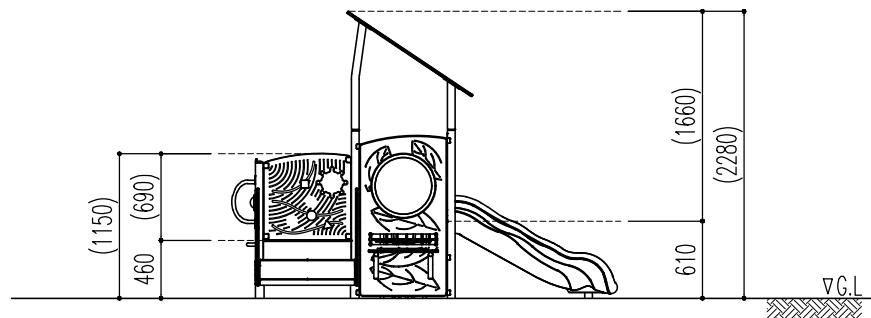
Y立面図 S=1:60
